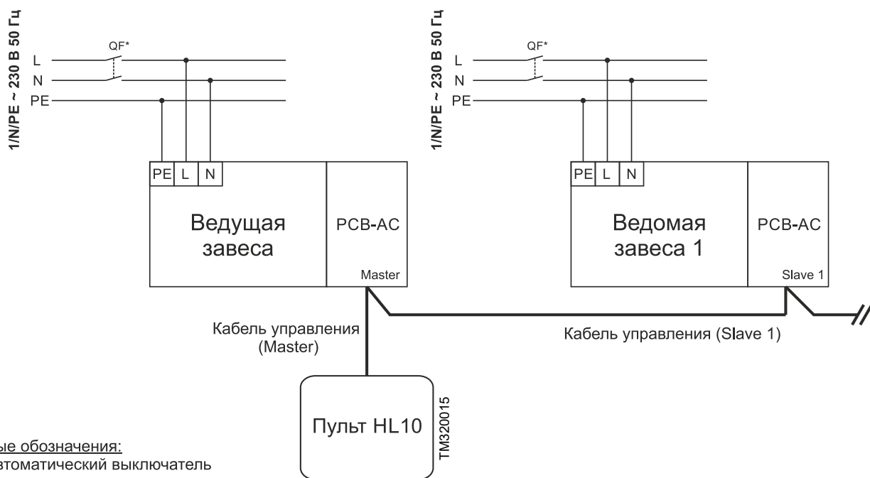
Схема подключения группы завес к однофазной сети переменного тока с напряжением ~ 230 В
